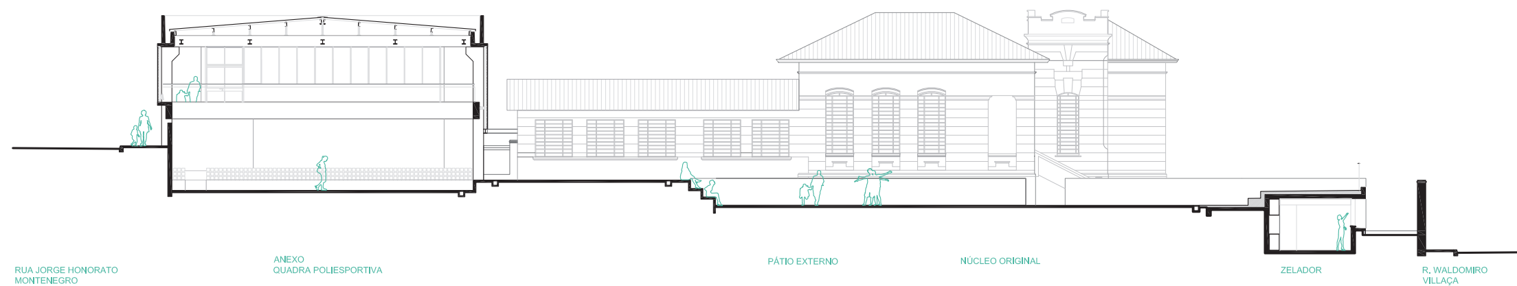
CORTE TRANSVERSAL PÁTIO LESTE 0 5m
