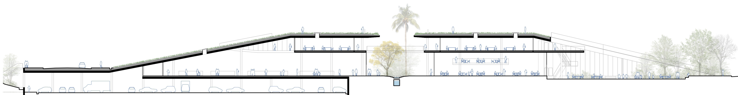
CORTE BOULEVARD ESC 1:500
