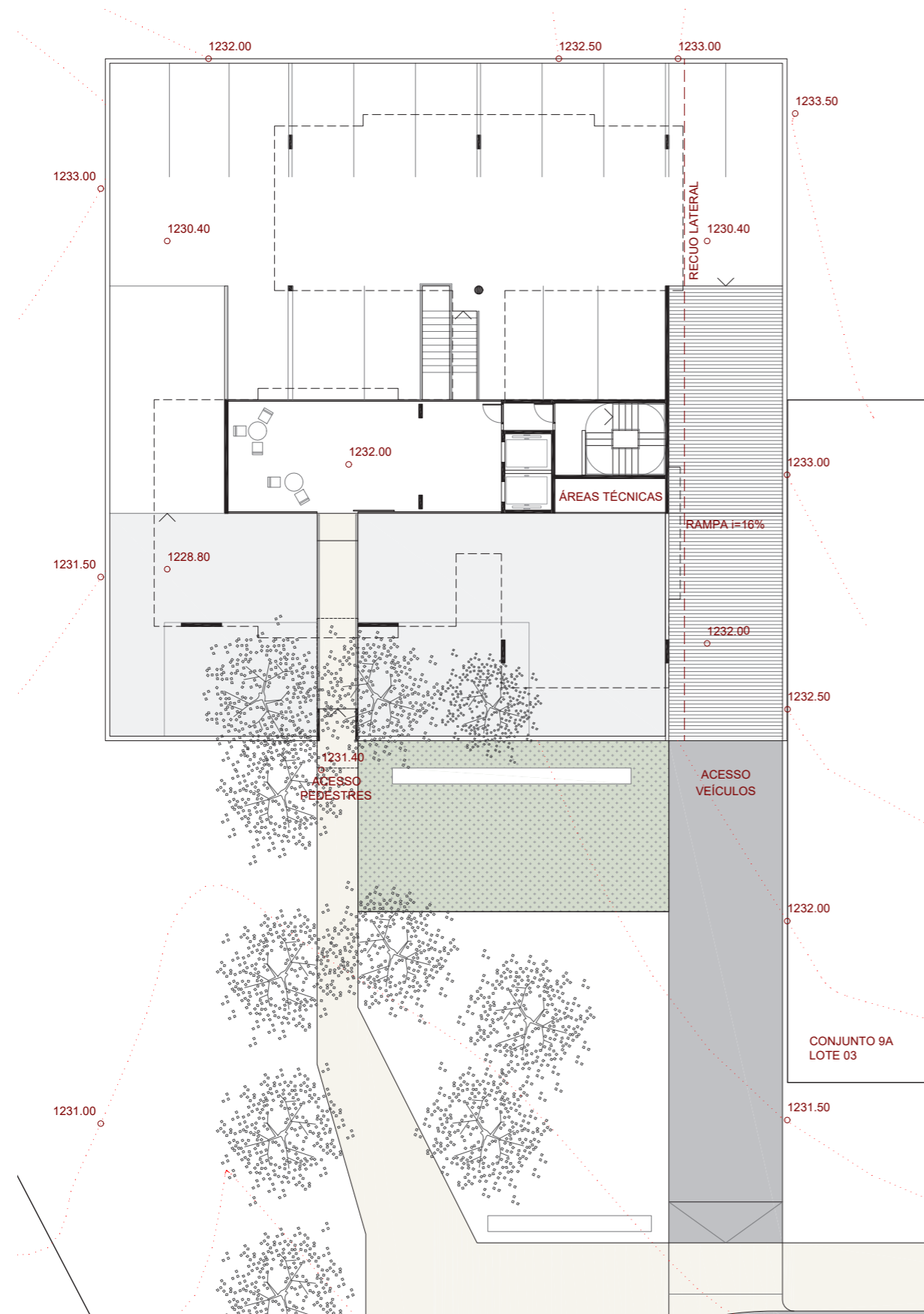
PLANTA TÉRREO/SEMI-SUBSOLO ESCALA 1:250
