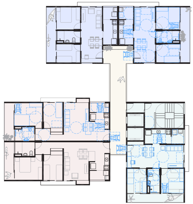
PAVIMENTO TIPO (1º ao 9º) ESCALA 1:125
