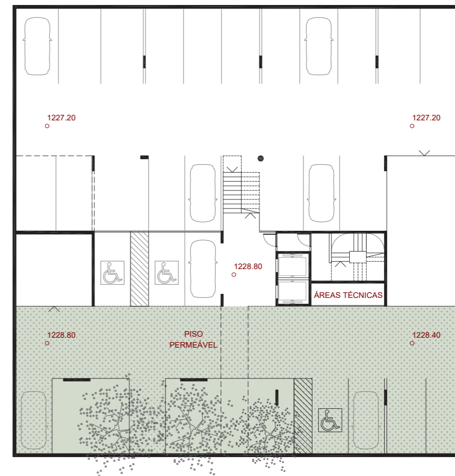
PLANTA SUBSOLO ESCALA 1:250
