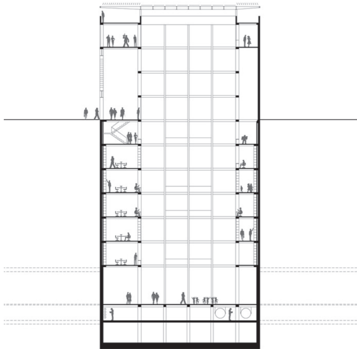
Corte Biblioteca
