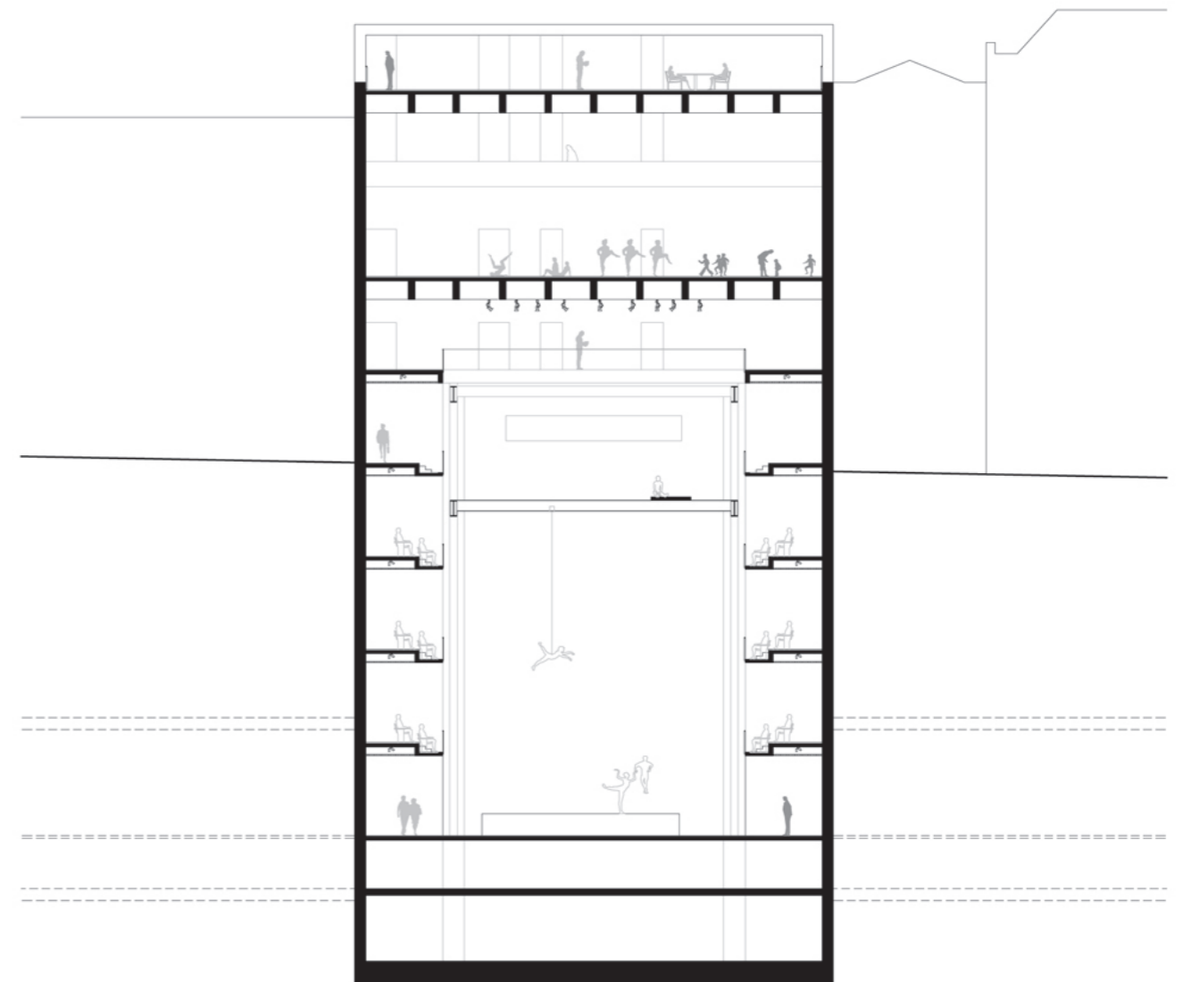
Corte Teatro
