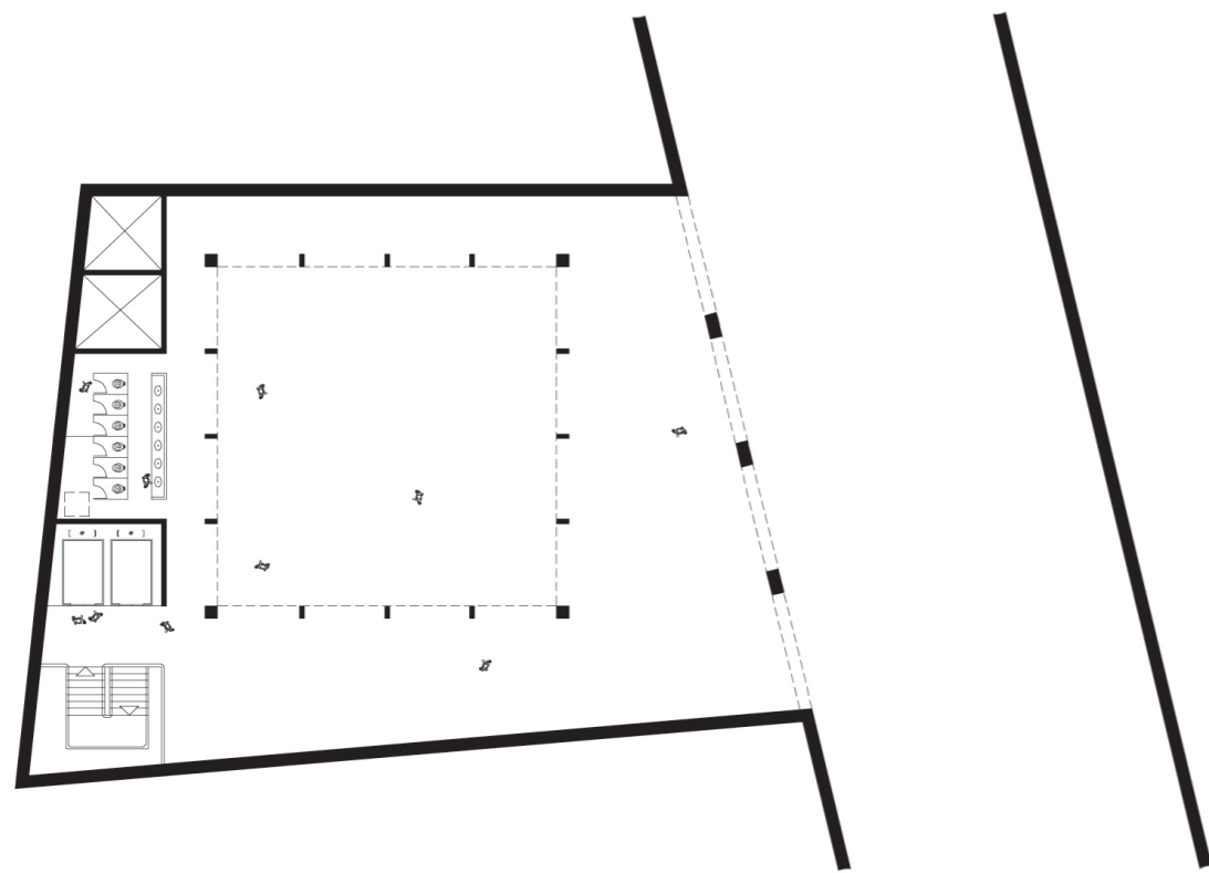
Planta Biblioteca - nível túnel
