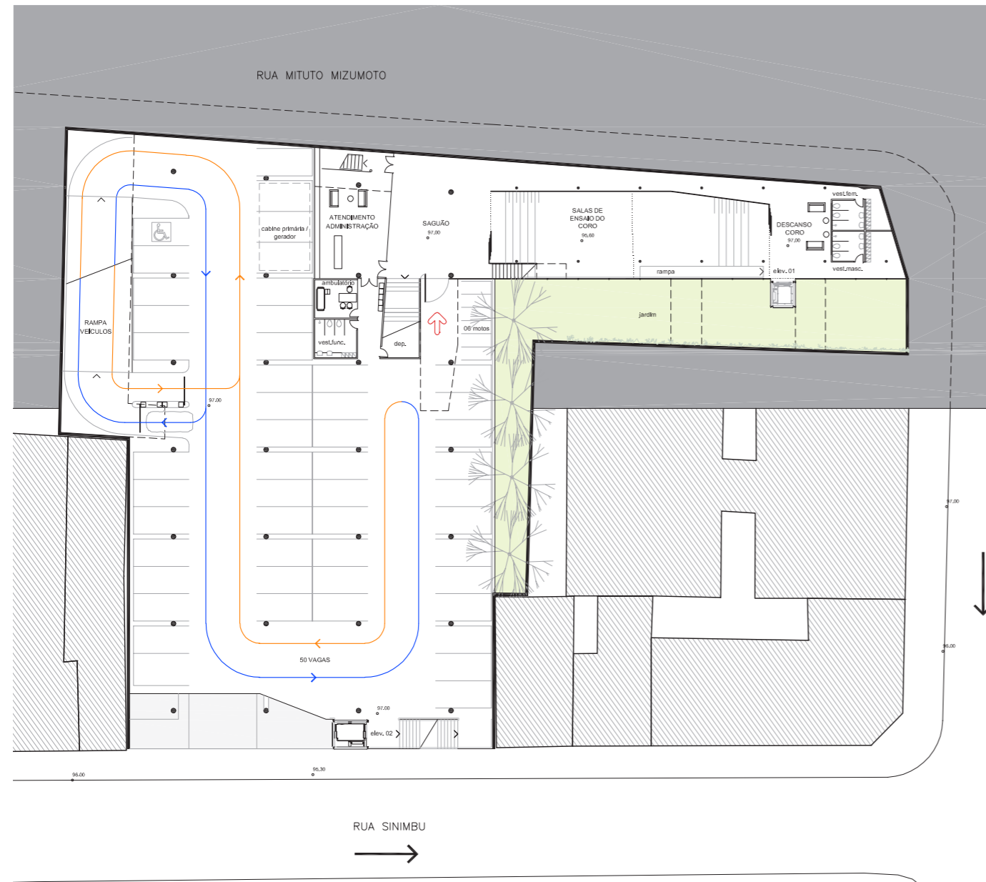
PLANTA PRIMEIRO SUBSOLO
