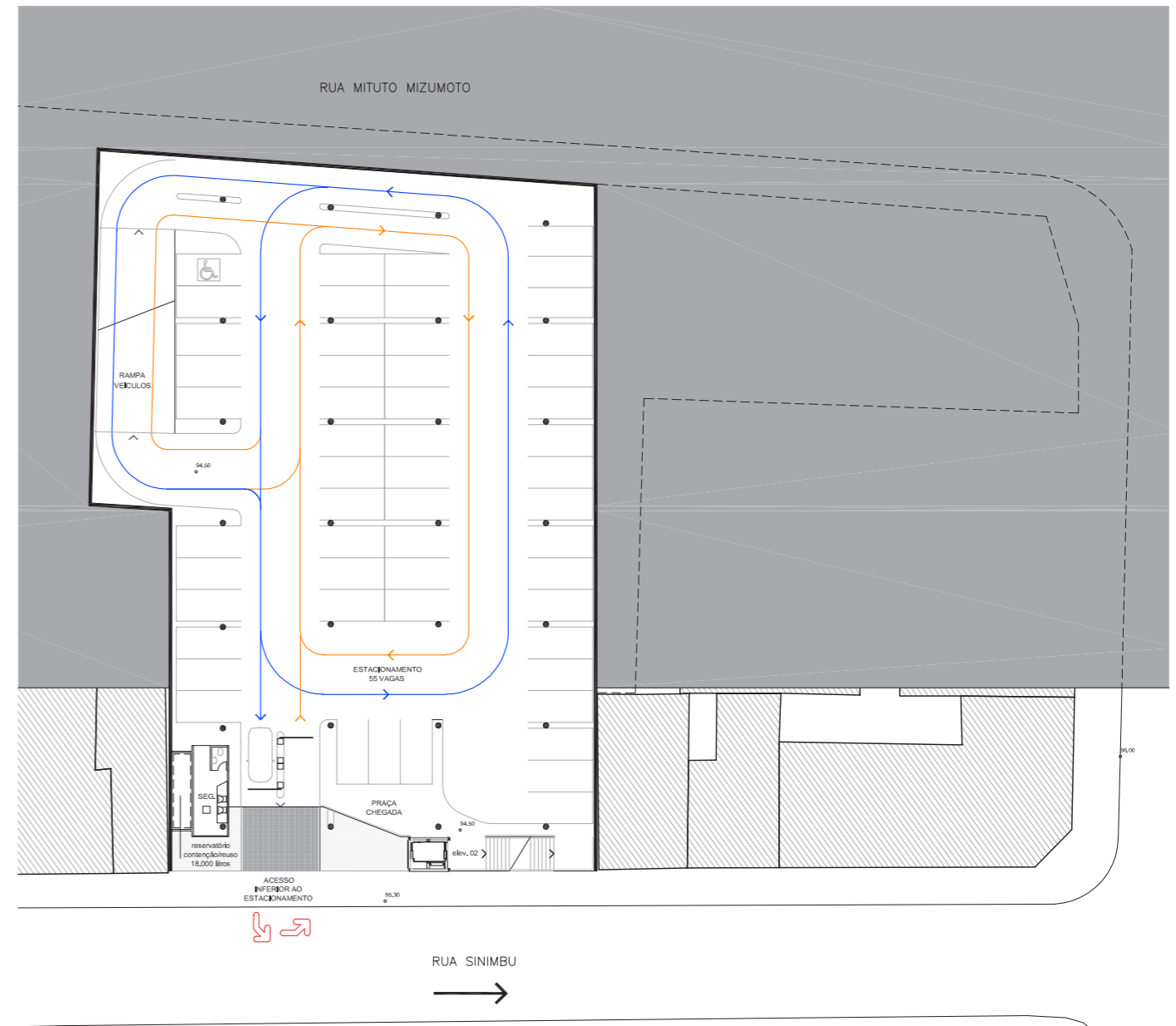
PLANTA SEGUNDO SUBSOLO
