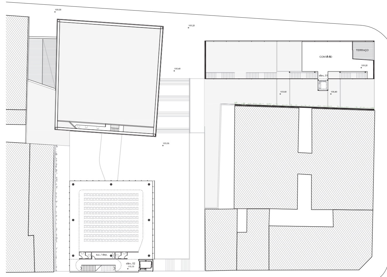
PLANTA SEGUNDO PAVIMENTO
