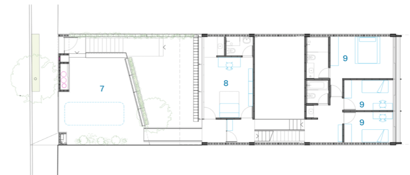
PLANTA DORMITÓRIOS
